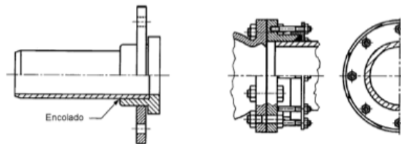
Figura 29 - Unión de brida
